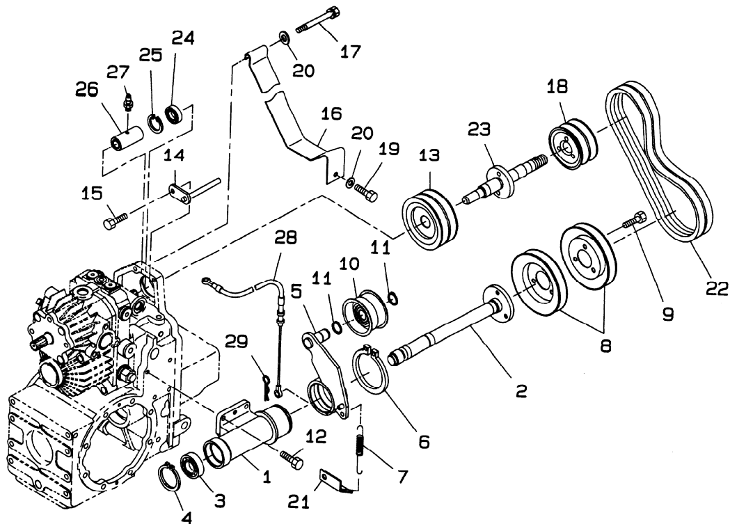
P.T.O;フロント FIG.222 POWER TAKE OFF;FRONT
