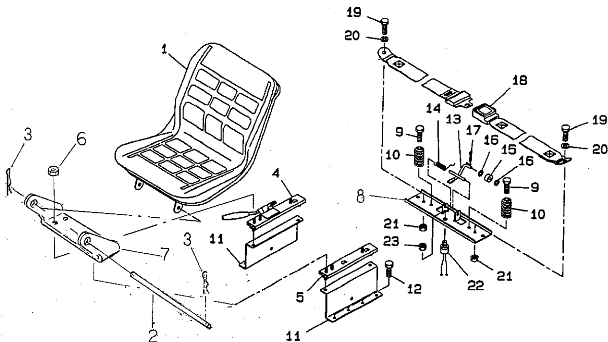
シート FIG.224 SEAT
