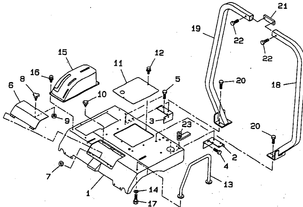
フエンダ&ROPS FIG.226 FENDER &ROPS
