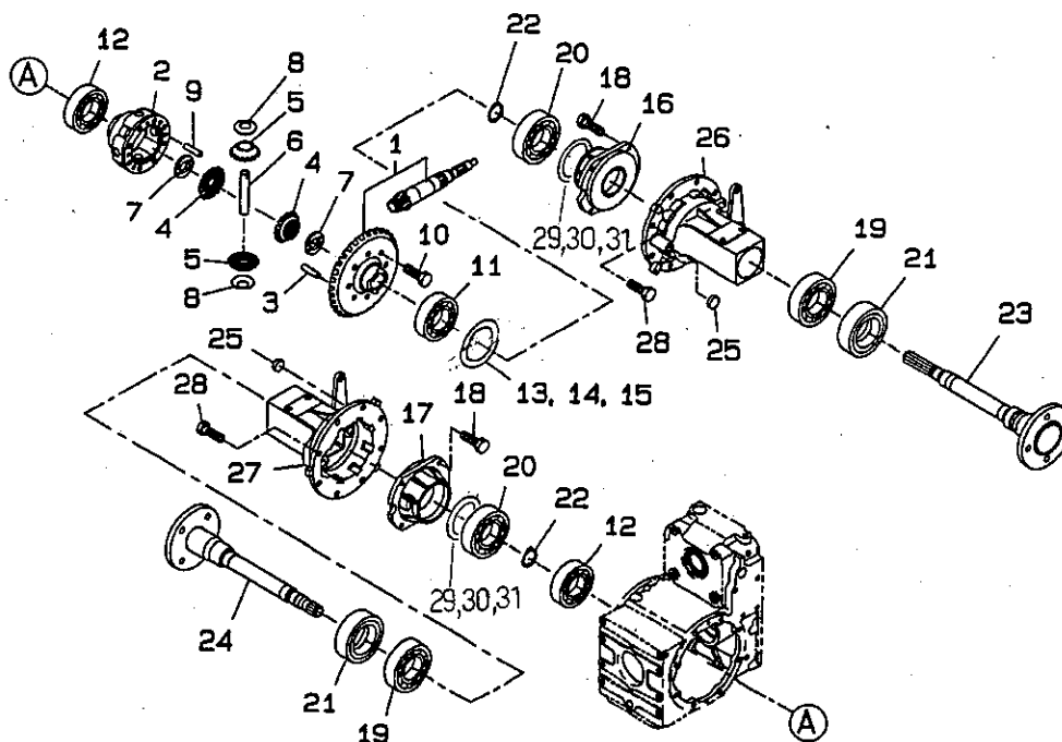
フロントデフ FIG.210 FRONT DIFFERENTIAL
