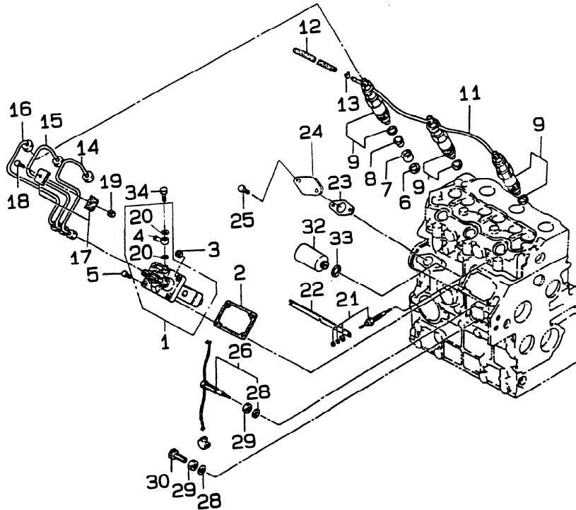
インジェクションポンプ FIG.108 INJECTION PUMP
