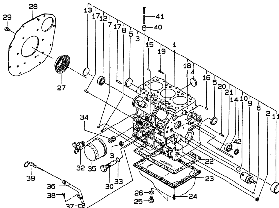
シリンダブロック FIG. 102 CYLINDER BLOCK
