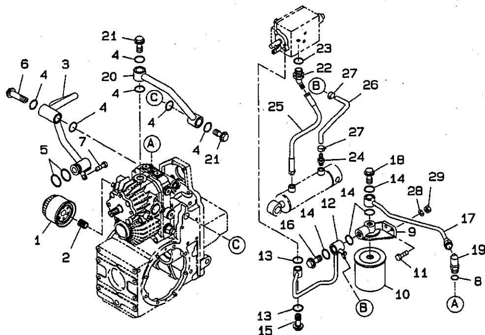
ユアツケイトウ;オイルフィルタ FIG.219 HYDRAULIC SYSTEM;OIL FILTER
