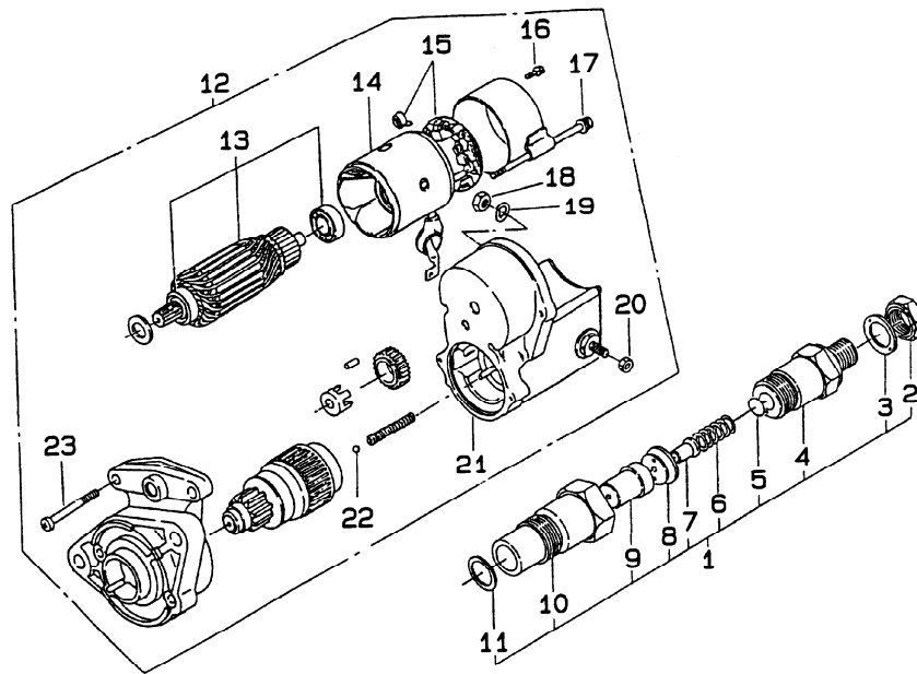
スターティングモータ,ノズル&ホルダ FIG.110 STARTING MOTOR,NOZZLE & HOLDER
