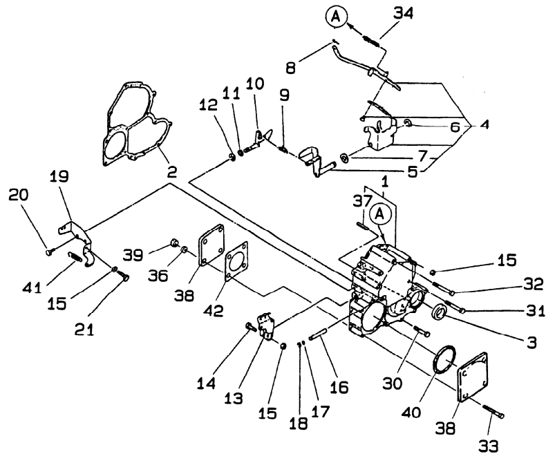
タイミングギヤケース FIG.107 TIMING GEAR CASE
