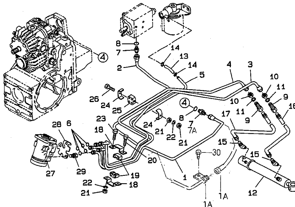
ユアツケイトウ;ステアリングケース FIG.218 HYDRAULIC SYSTEM;STEERING CASE
