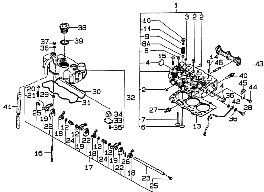
シリンダヘッド FIG. 103 CYLINDER HEAD
