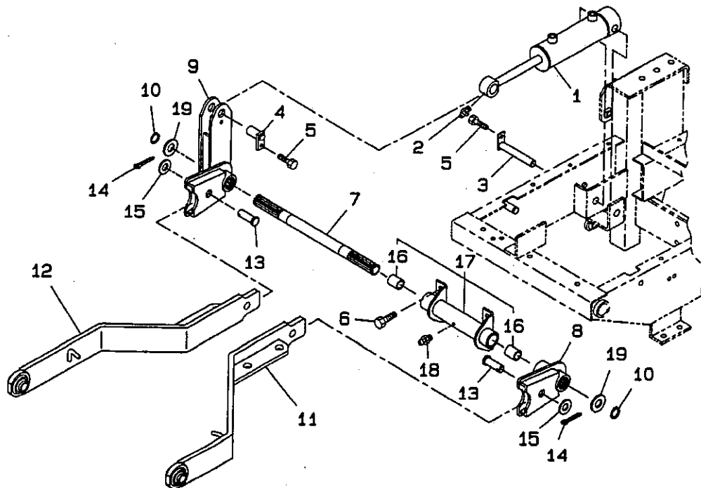
リフトリンク FIG.207 LIFT LINKAGES
