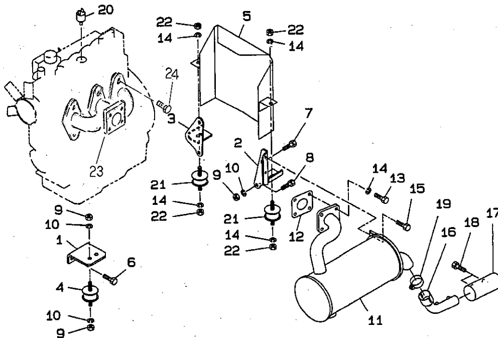
マフラ,エンジンマラント FIG.203 MUFFLER,ENGINE MOUNT
