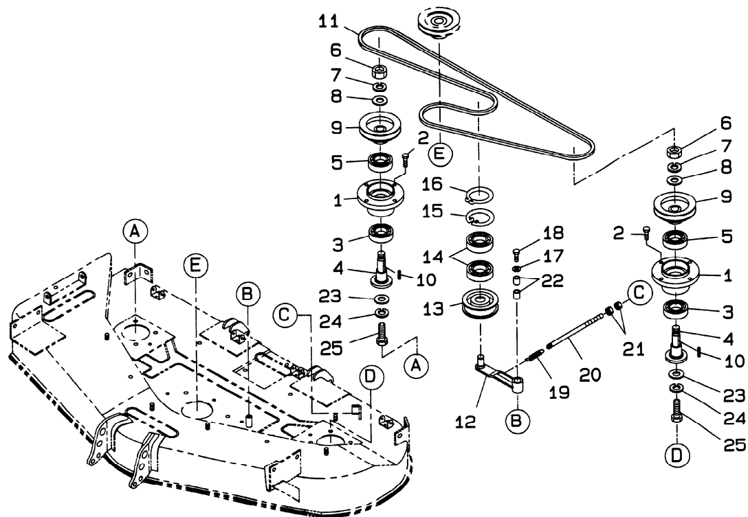
プーリ;48インチ モア FIG.302 PULLEY;48 INCH MOWER
