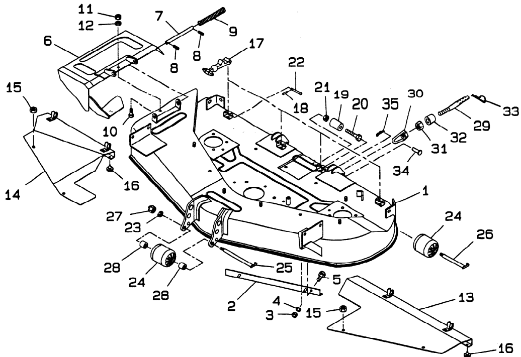
モアデツキ;48インチ モア FIG.303 MOWER DECK;48INCH MOWER
