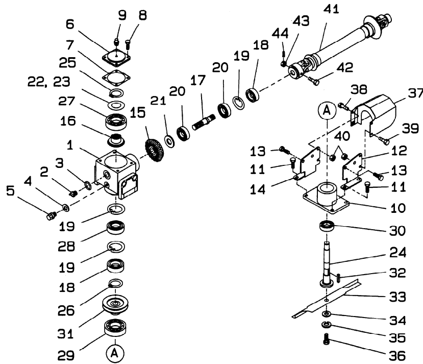
ギヤボックス;48インチ モア FIG.301 GEAR BOX;48INCH MOWER
