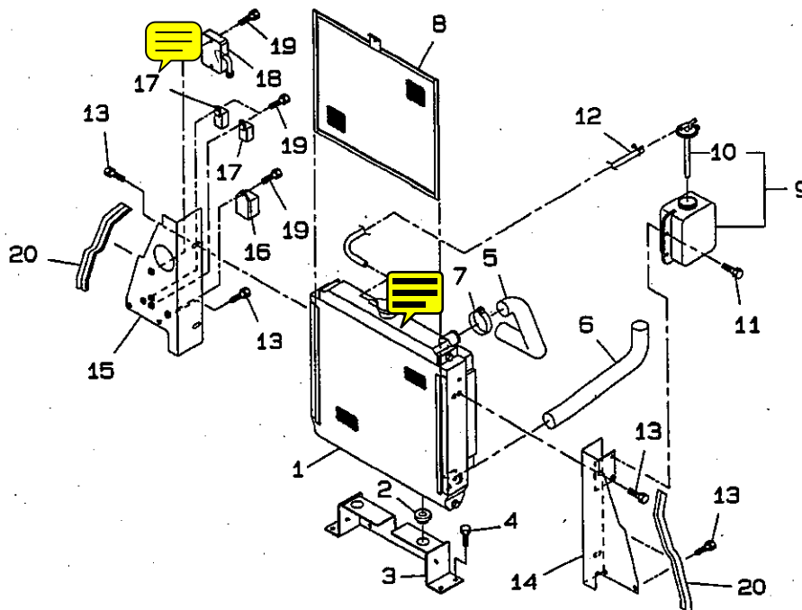
ラジエータ FIG.205 RADIATOR
