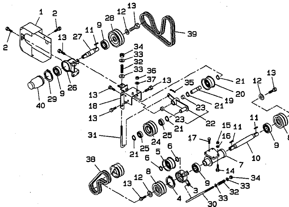
P.T.O;サイド FIG.221 POWER TAKE OFF;SIDE
