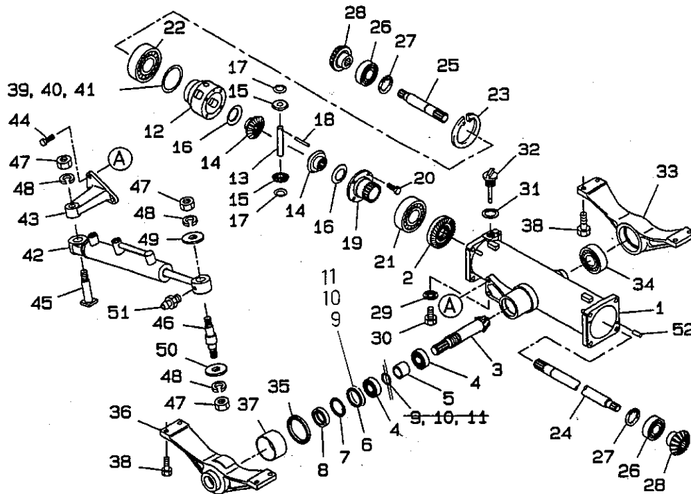
リヤアデフアレンシャル FIG.211 REAR DIFFERENTIAL
