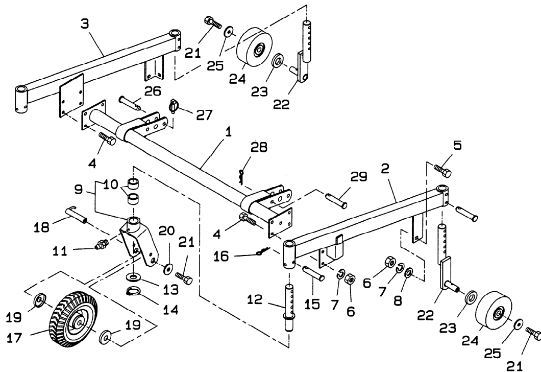
ゲージホイール;48インチ モア FIG.304 GAUGE WHEEL;48INCH MOWER
