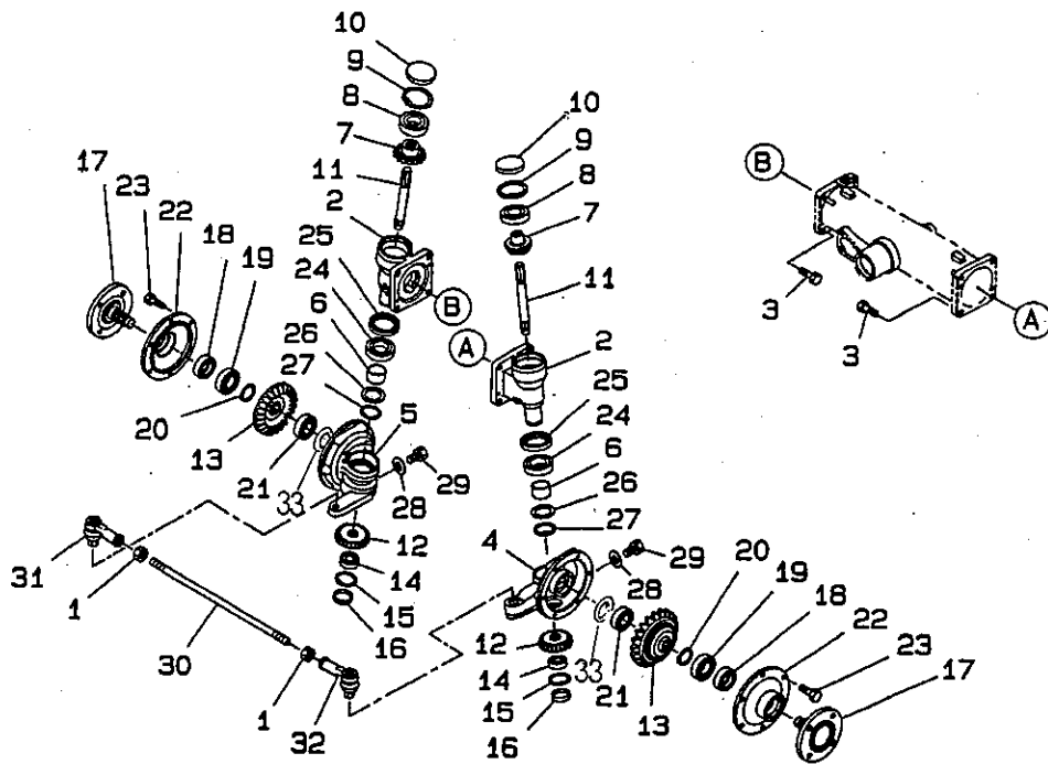
リヤアスクル FIG.212 REAR AXLE
