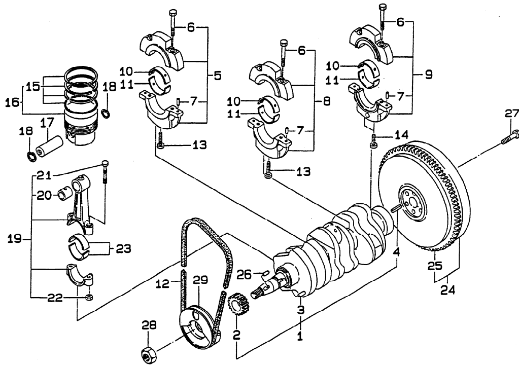
クランクシャフト FIG. 104 CRANK SHAFT
