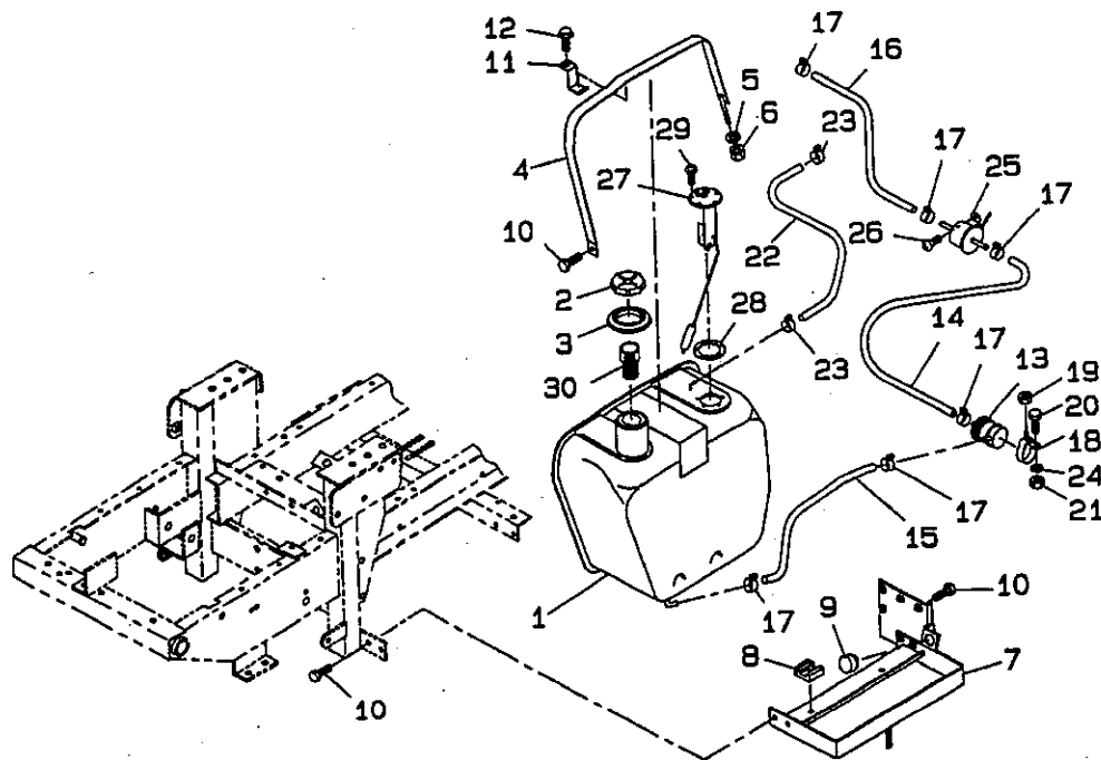
フュエルタンク FIG.202 FUEL TANK
