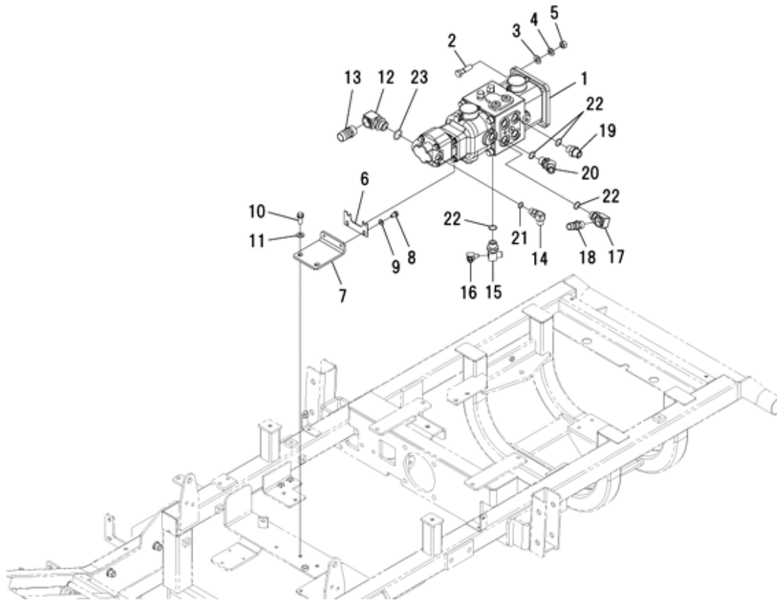
FIG.218 ユアツ ; HST HYDRAULIC ; HST
