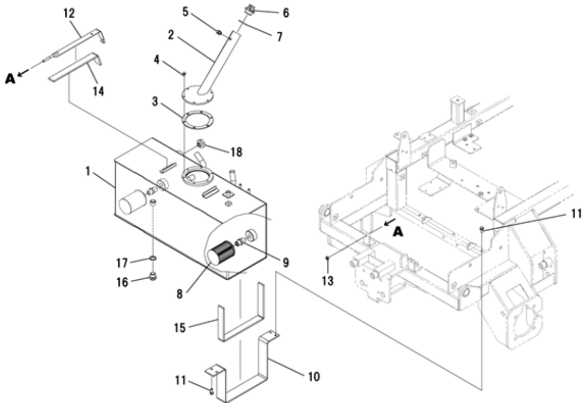
FIG.203 オイルタンク OIL TANK
