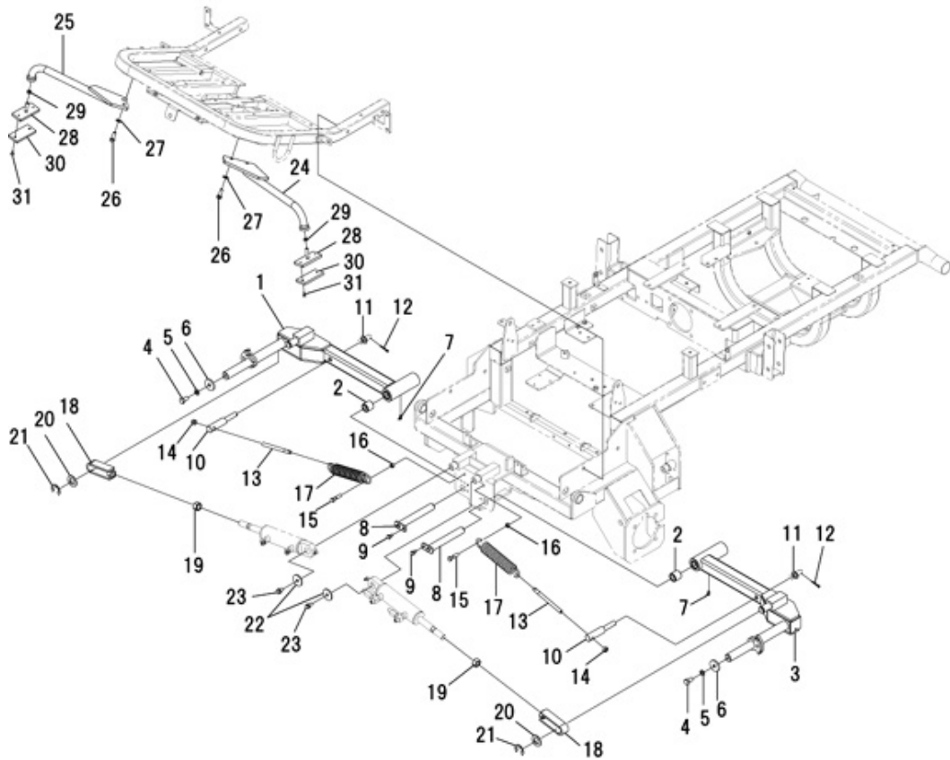
FIG.211 カッターアーム；フロント CUTTER ARM ; FRONT
