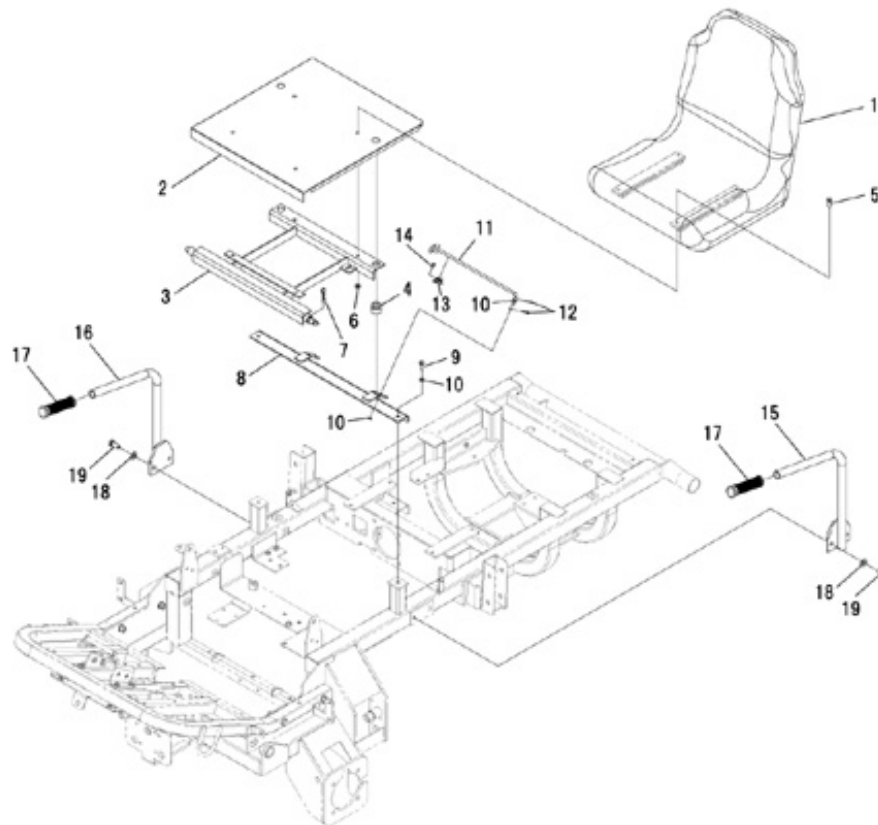
FIG.215 シート SEAT
