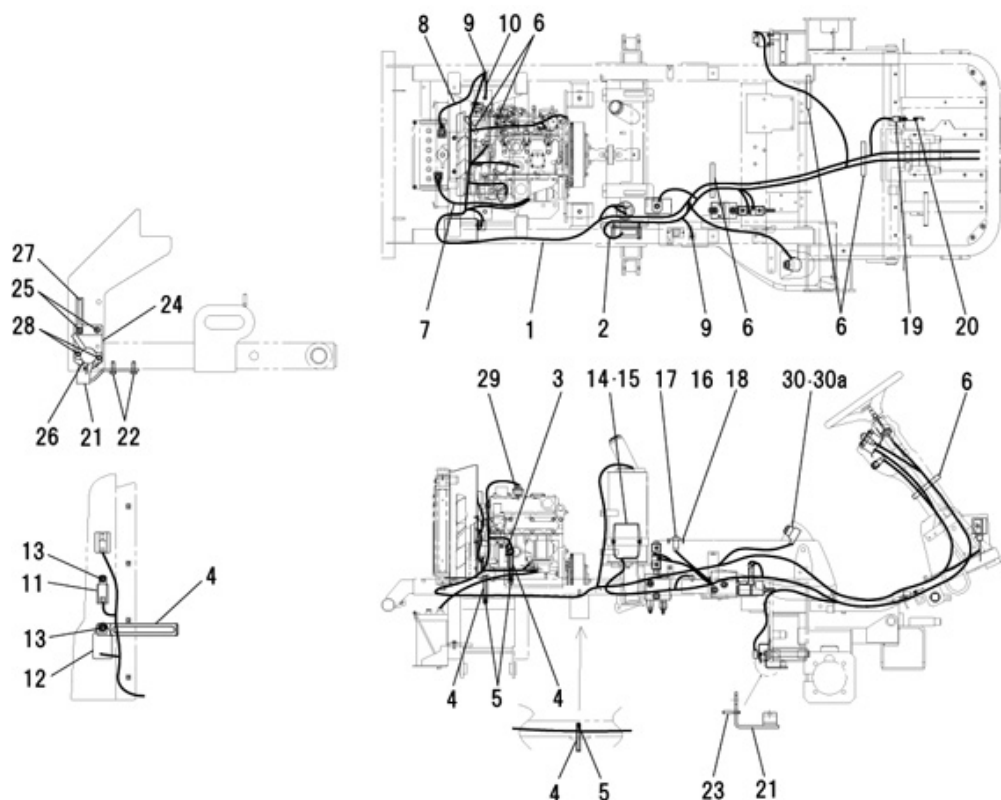
ワイヤハーネス FIG.228 WIRE HARNESS
