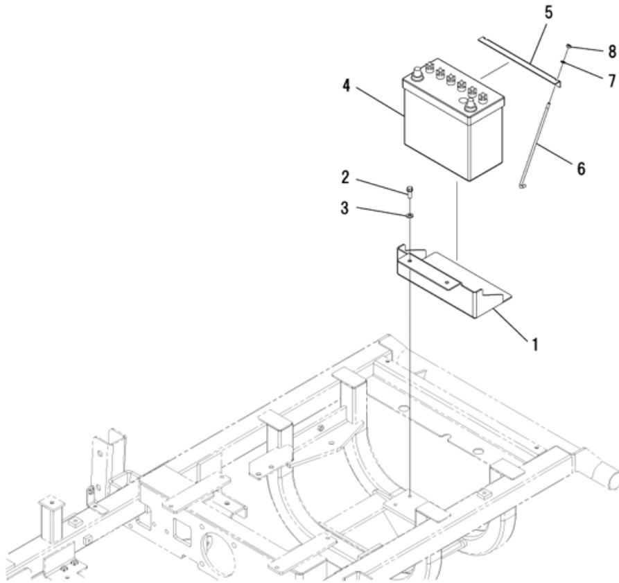
バッテリー BATTERY
