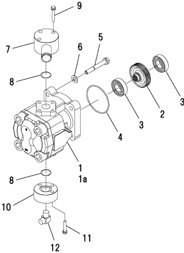
ポンプ PUMP
