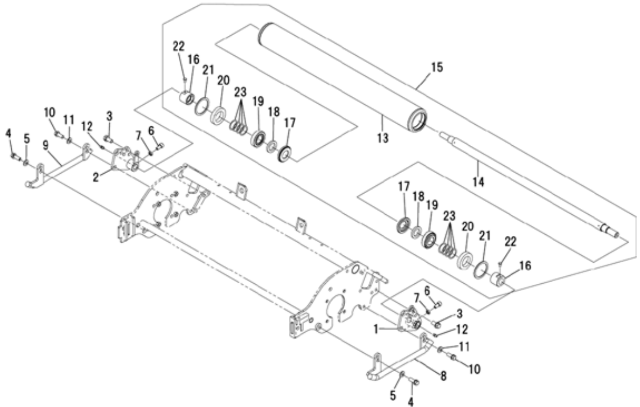
FIG.304 リヤローラ REAR ROLLER
