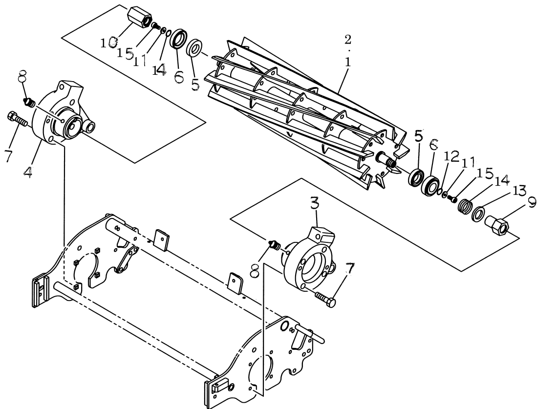
FIG.302 リールブレード REEL BLADE
