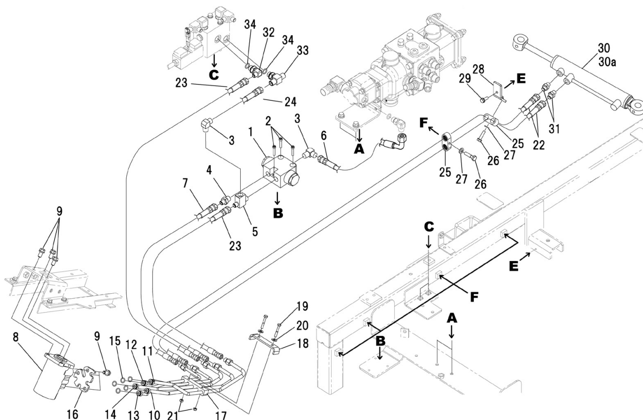
FIG.220 ユアツ；ステアリング HYDRAULIC ; STEERLING
