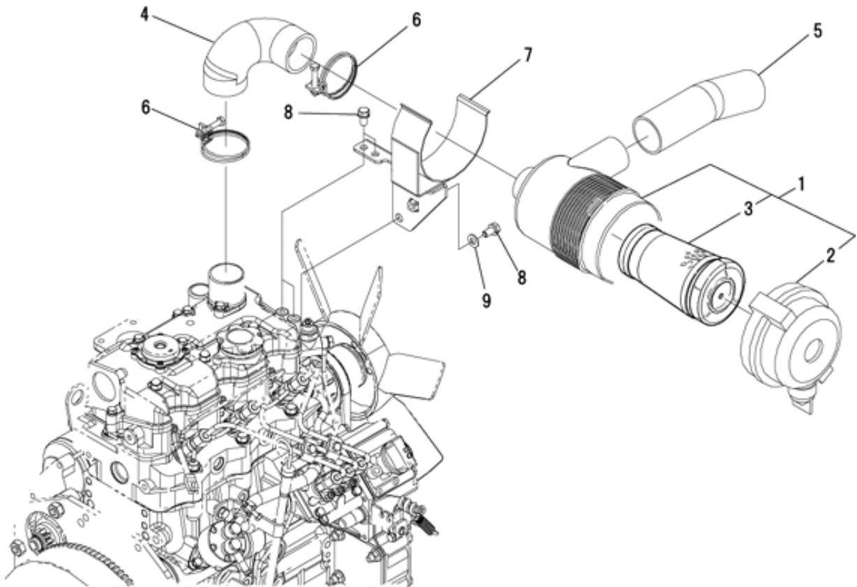
エアクリーナ AIR CLEANER
