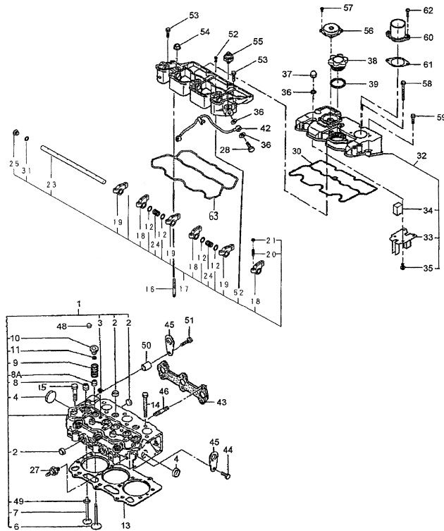
シリンダ ヘッド FIG.103 CYLINDER HEAD
